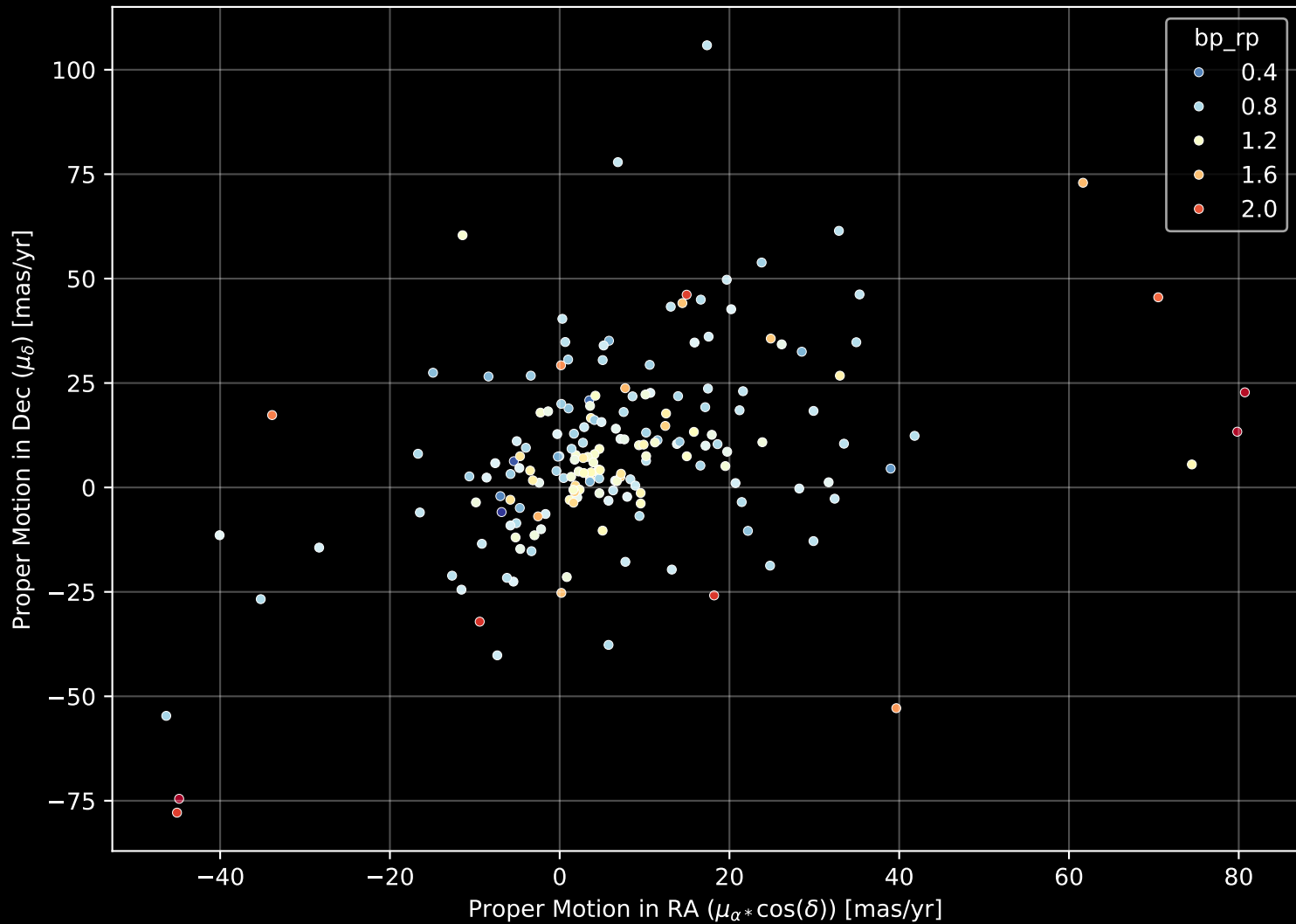
APOGEE DR17 Field: [281-39-O_TESS] Proper Motion Diagram (n= 186)
