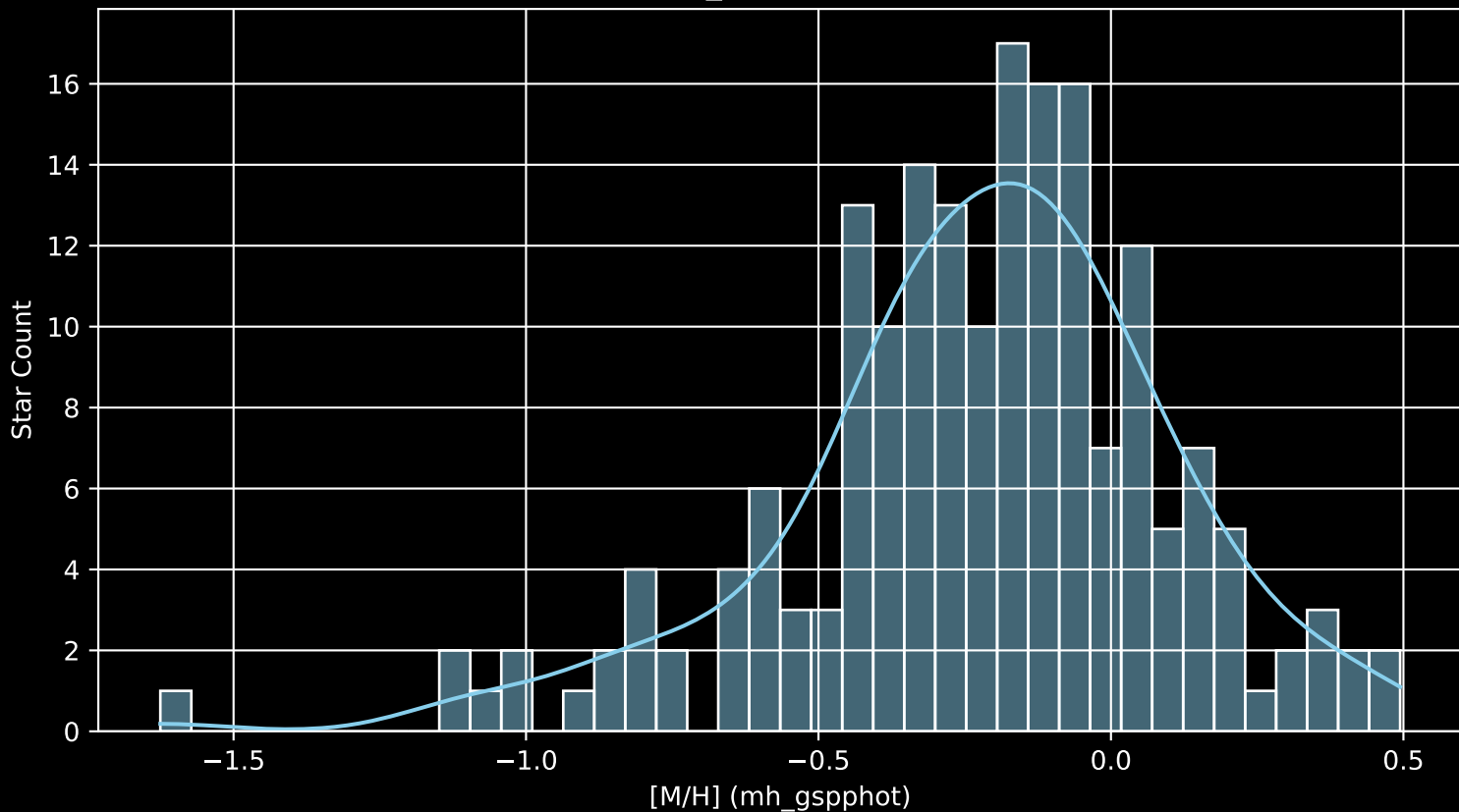
APOGEE DR17 Field: [281-39-O_TESS [M/H] (mh_gspphot) (n= 186)
