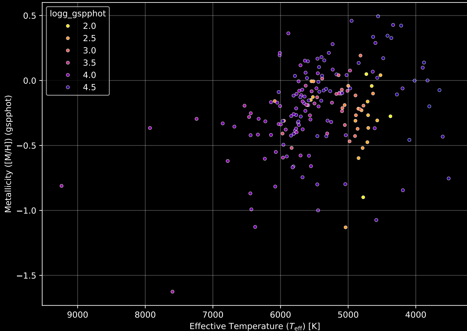
APOGEE DR17 Field: [281-39-O_TESS] Stellar Population Parameters (n= 186)
