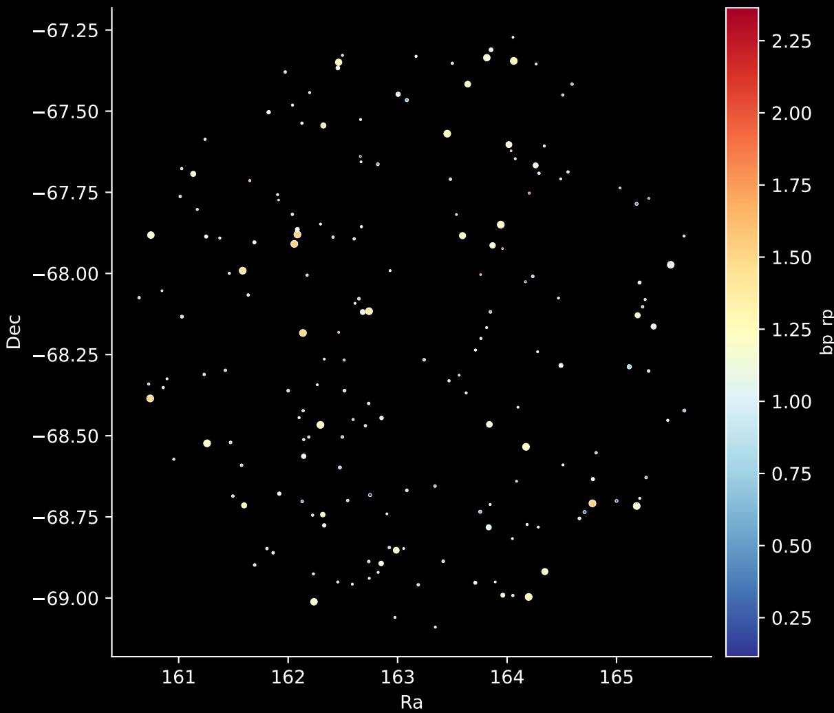
APOGEE DR17 Field: [281-39-O_TESS] Stars: 186
